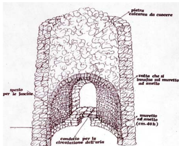
Schema di calchèra.
